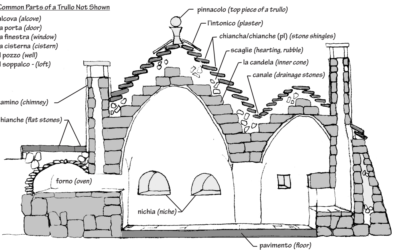
Parts Of A Trullo / Componenti Del Trullo
